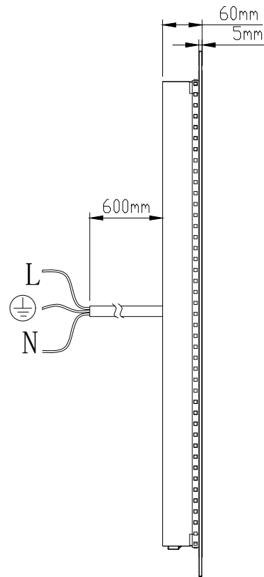
LEFT SIDE
